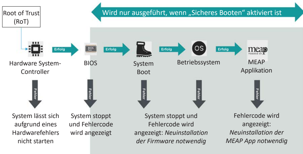
Abbildung 3 Prozess der Systemüberprüfung beim Systemstart
