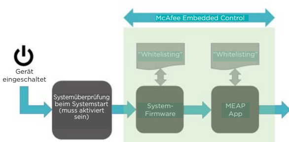
Abbildung 4 Bootprozess des Systems ab Start und während der Laufzeit
