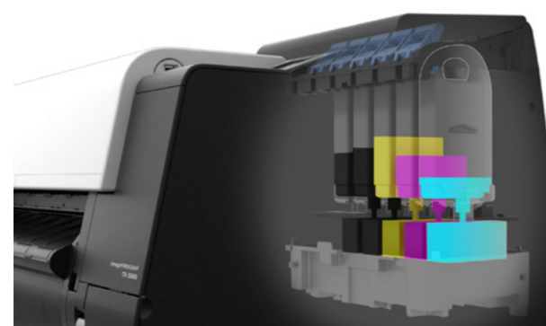
Les réservoirs d'encre secondaires permettent une impression continue lors du remplacement des cartouches d'encre
