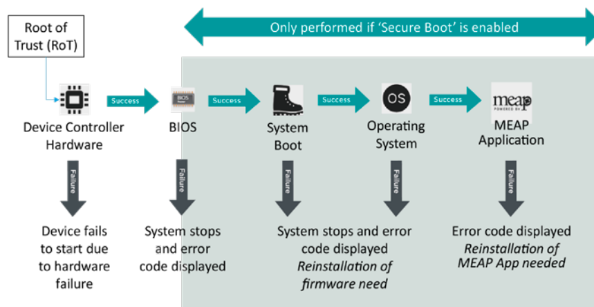
Abbildung 3 Prozess der Systemüberprüfung beim Systemstart
