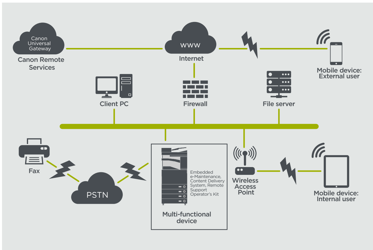
Abbildung 9 Verteilte Verbindung
