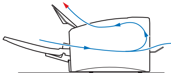
Standard- und gerader Papierweg
